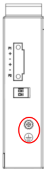
Рисунок 4 — Винт заземления на коммутаторе
