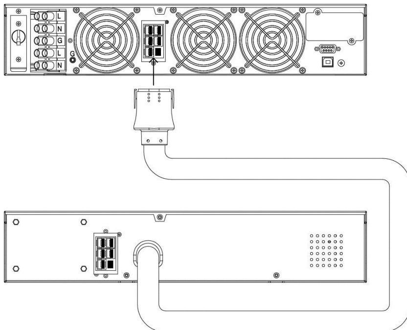
Рис. 4. Подключение внешнего батарейного блока
